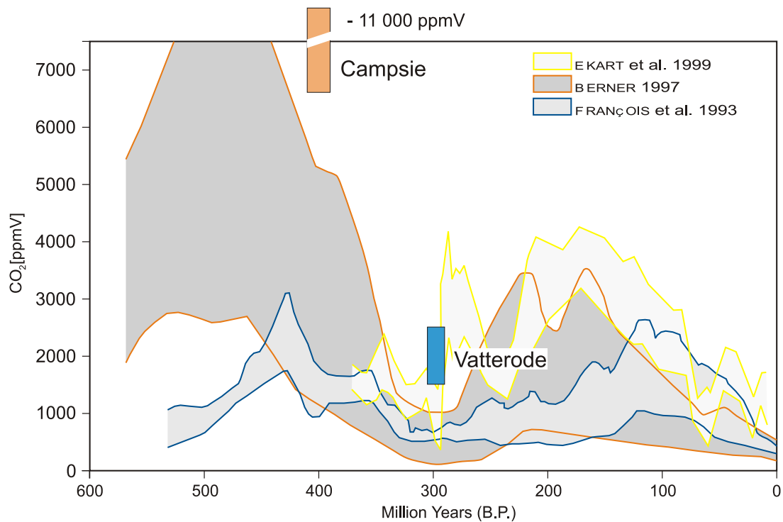
Abb. 42: Aus den Isotopendaten der Lokalitäten Campsie und Vatterode ermittelte \text{CO}_2 -Konzentrationen in der Paläoatmosphäre im Vergleich mit modellierten \text{CO}_2 -Gehalten.
