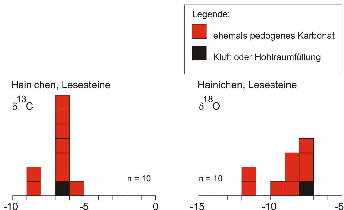
Abb. 37: Verteilung der C- und O-Isotopenwerte in Leseproben der Lokalität Hainichen.
