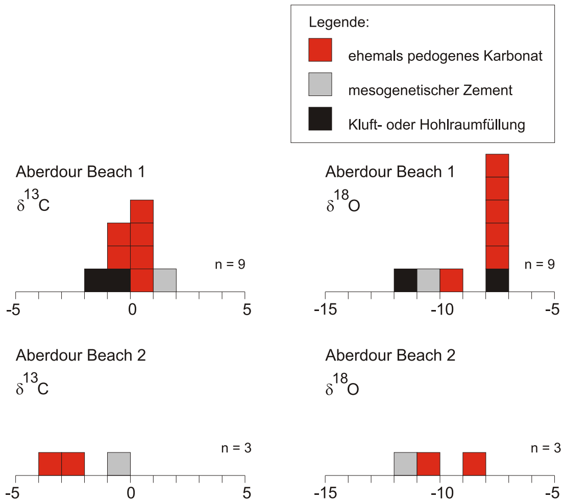
Abb. 26: Verteilung der C- und O-Isotopenwerte in den Profilen der Lokalität Carnoustie.
