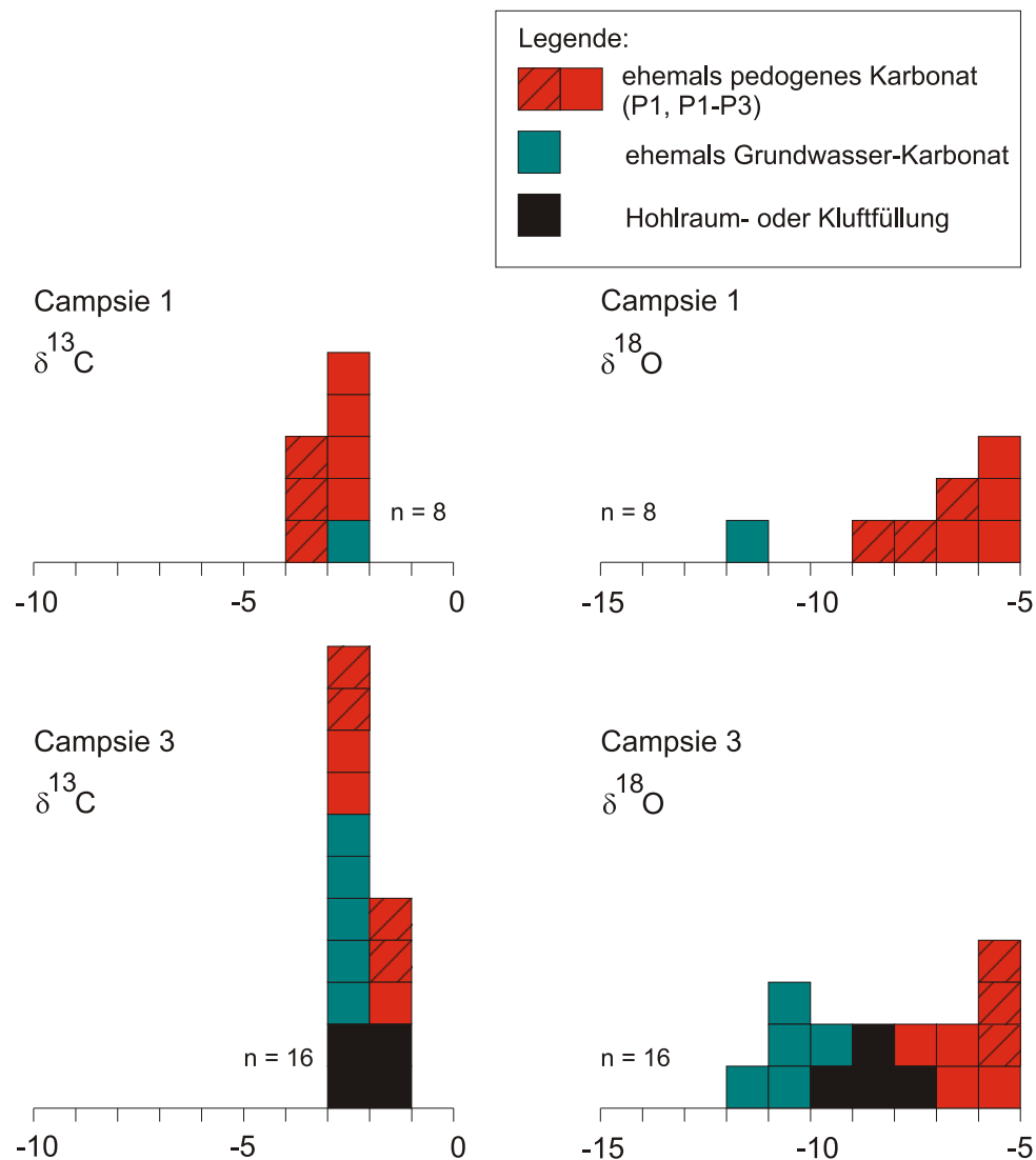
Abb. 24: Verteilung der C- und O-Isotopenwerte in den einzelnen Profilen der Lokalität Campsie.
