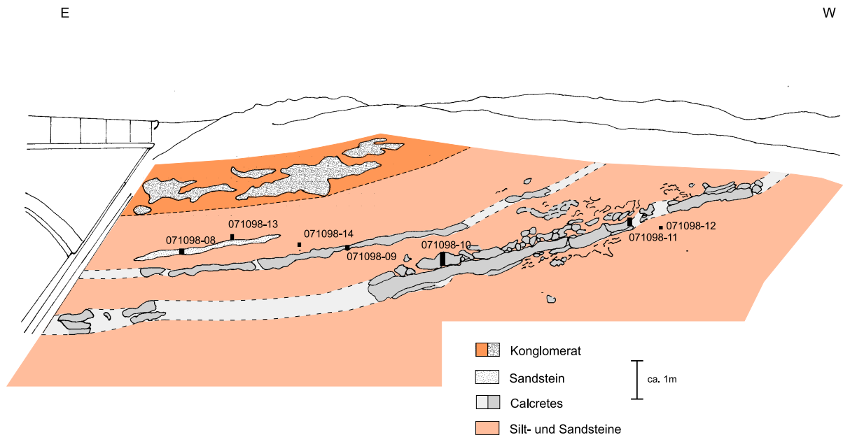
Abb. 17: Oberer Teil (Abschnitt 3) des aufgenommenen Profils am Bahnanschnitt Vatterode, westlich der Fußgängerbrücke, mit eingetragenen Probenahmepunkten
