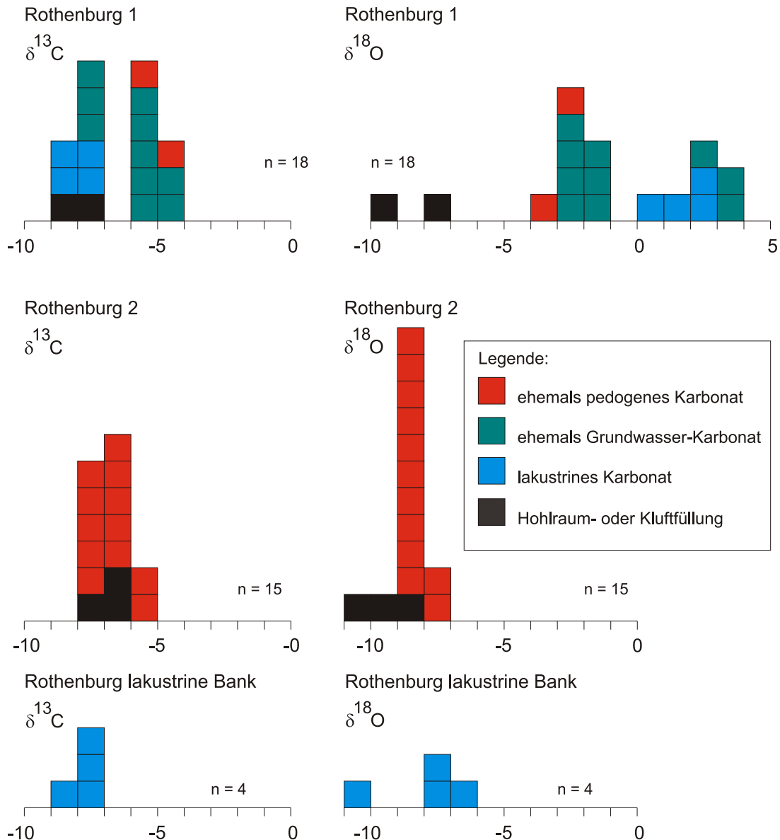
Abb. 34: Verteilung der C- und O-Isotopenwerte in den Profilen der Lokalität Rothenburg.
