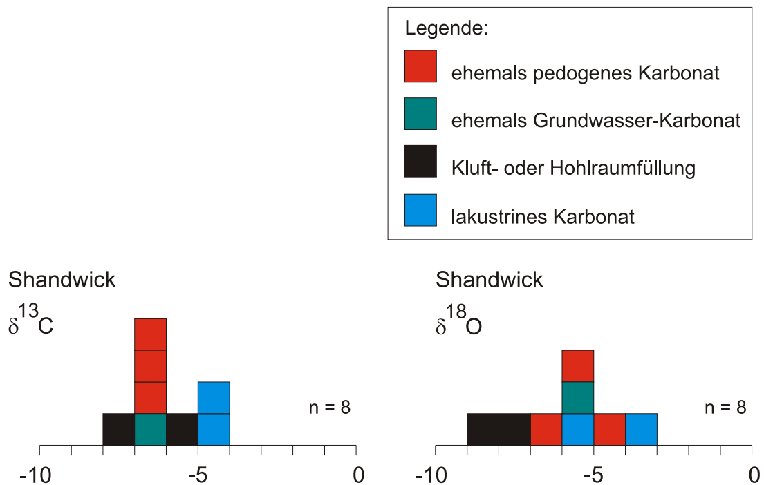
Abb. 28: Verteilung der C- und O-Isotopenwerte im Profil 2 der Lokalität Shandwick.
