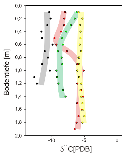
Abb. 43: Tiefenverteilung von \delta^{13}\text{C} -Werten in einer Bodenbildung im Profil Vatterode. Tiefenverteilung von \delta^{13}\text{C} -Werten in rezenten Bodenbildungen, nach verschiedenen Bearbeitern.
