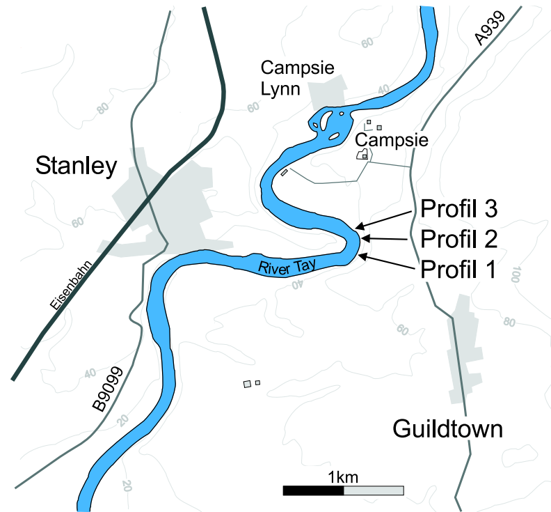
Abb. 13: Lage der Profile Campsie 1-3 am Ufer des Tays südlich von Campsie
