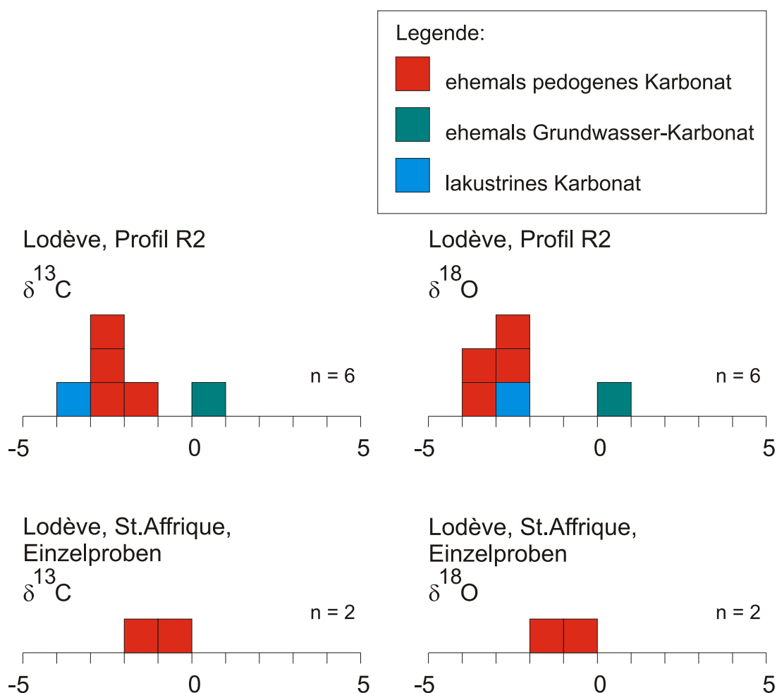
Abb. 39: Verteilung der C- und O-Isotopenwerte im Profil R2 der Lokalität Lodève und in Einzelproben aus dem Lodève- und St. Affrique-Becken.
