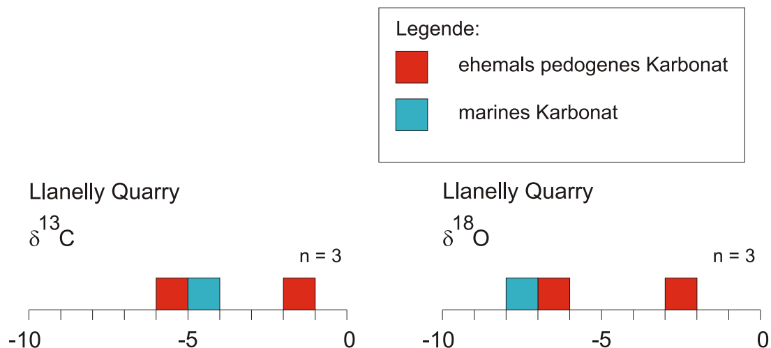
Abb. 32: Verteilung der C- und O-Isotopenwerte im Profil der Lokalität Llanelly Quarry.
