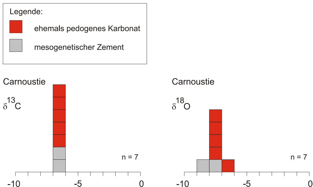
Abb. 25: Verteilung der C- und O-Isotopenwerte im Profil der Lokalität Carnoustie.
