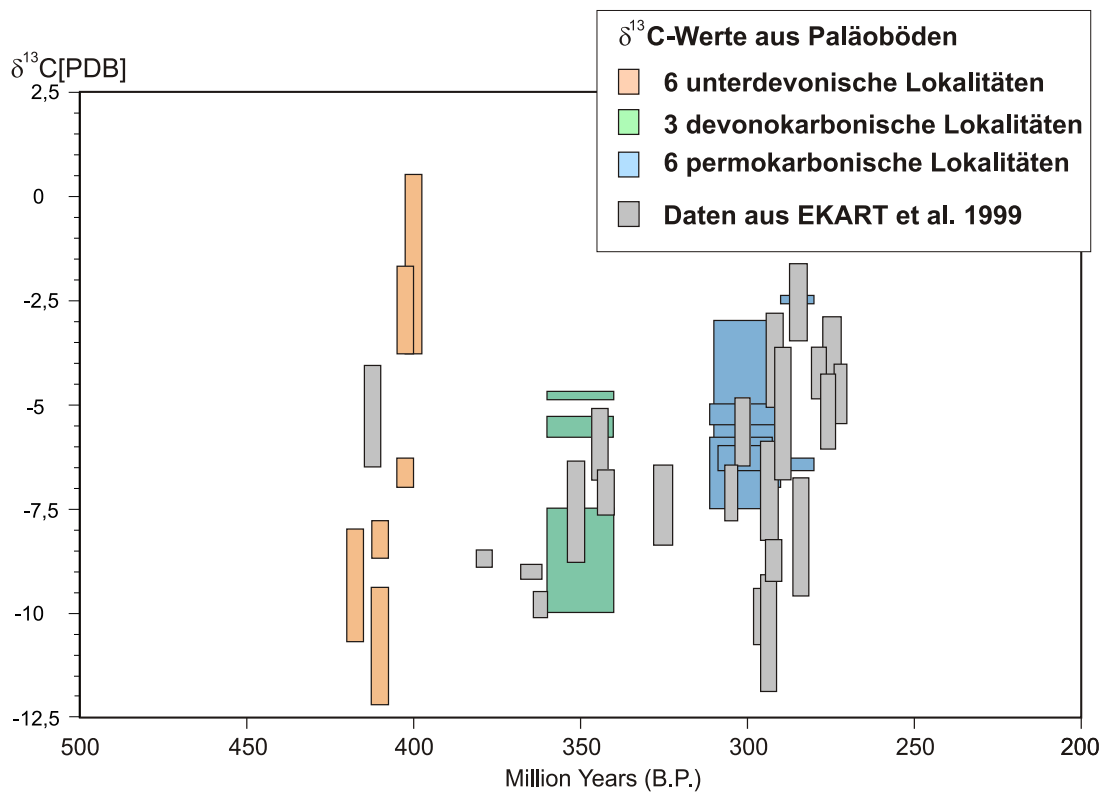
Abb. 41: \delta^{13}\text{C} -Werte aus den untersuchten Lokalitäten mit Bodenbildungen. Im Vergleich Literaturwerte aus EKART et al. 1999
