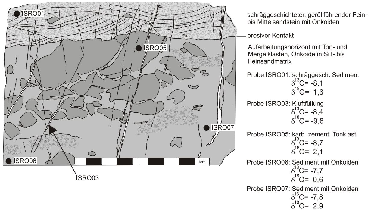
Abb. 19: Handstück 111198-4 aus der Kalksteinbank des Profils Rothenburg 1, mit eingetragenen Probenahmestellen für die Isotopenbestimmungen.
