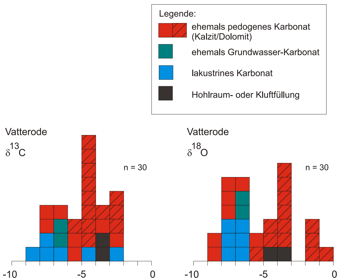
Abb. 33: Verteilung der C- und O-Isotopenwerte im Profil der Lokalität Vatterode.
