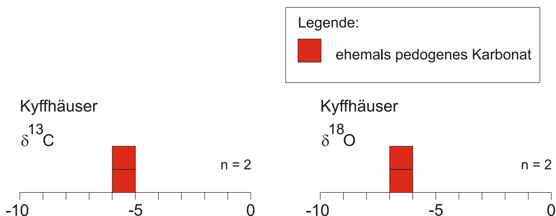
Abb. 36: Verteilung der C- und O-Isotopenwerte im Profil der Lokalität Kyffhäuser.
