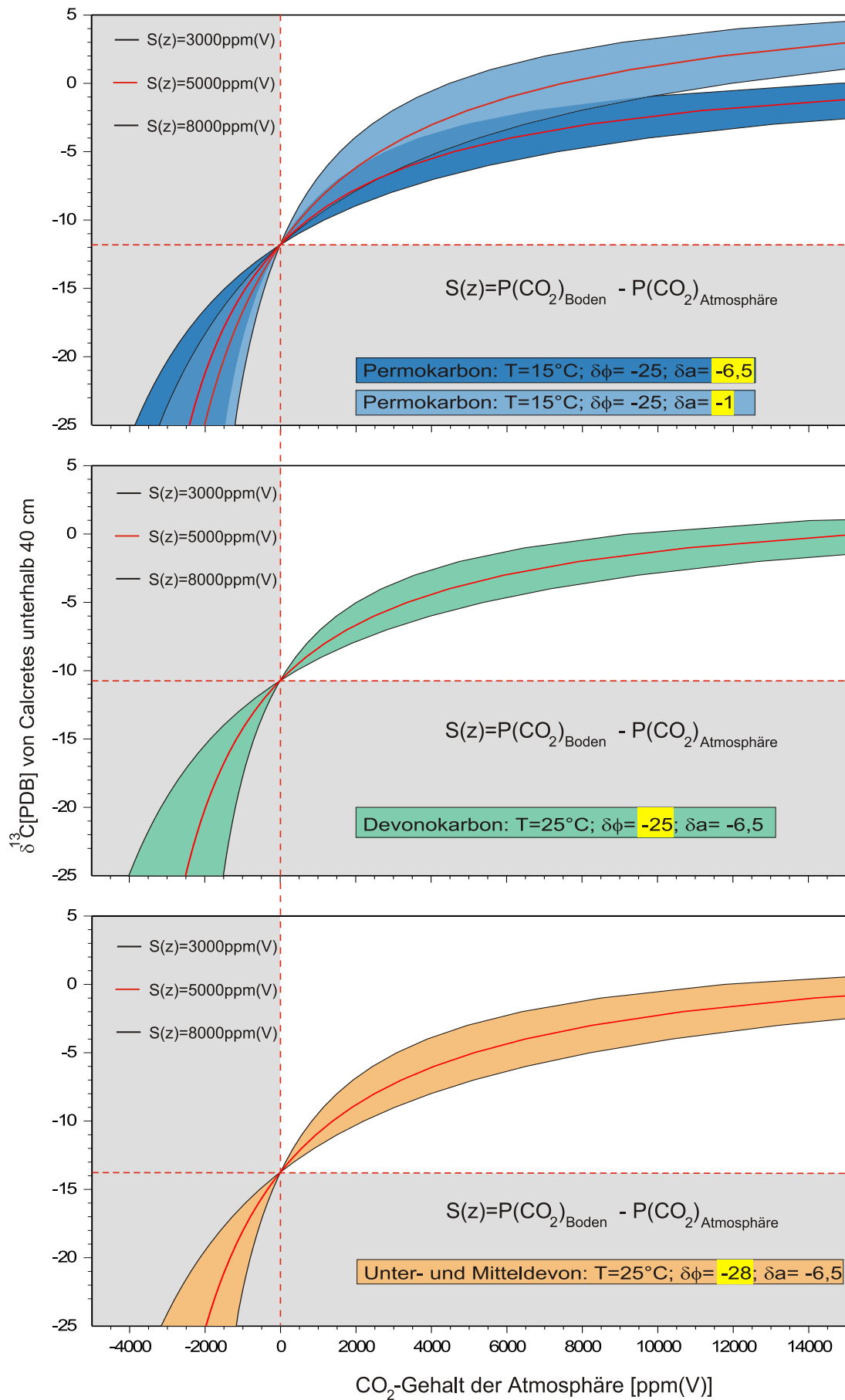
Abb. 5: Modelle nach CERLING (1991,1999). Erläuterungen s. Text.
