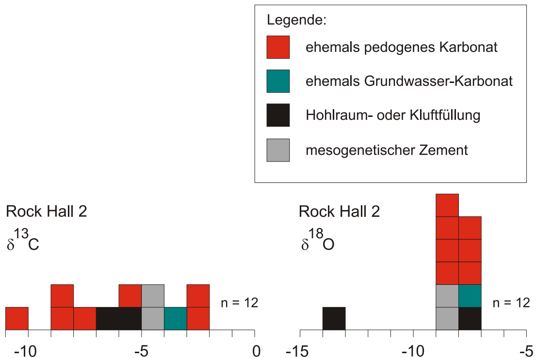
Abb. 31: Verteilung der C- und O-Isotopenwerte im Profil 2 der Lokalität Rock Hall.
