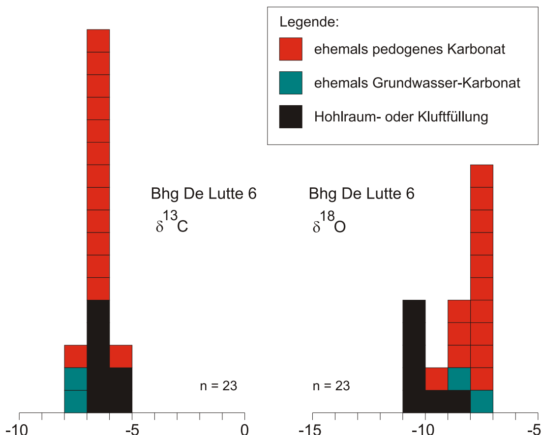
Abb. 38: Verteilung der C- und O-Isotopenwerte in Kernabschnitten der Bohrung De Lutte 6.
