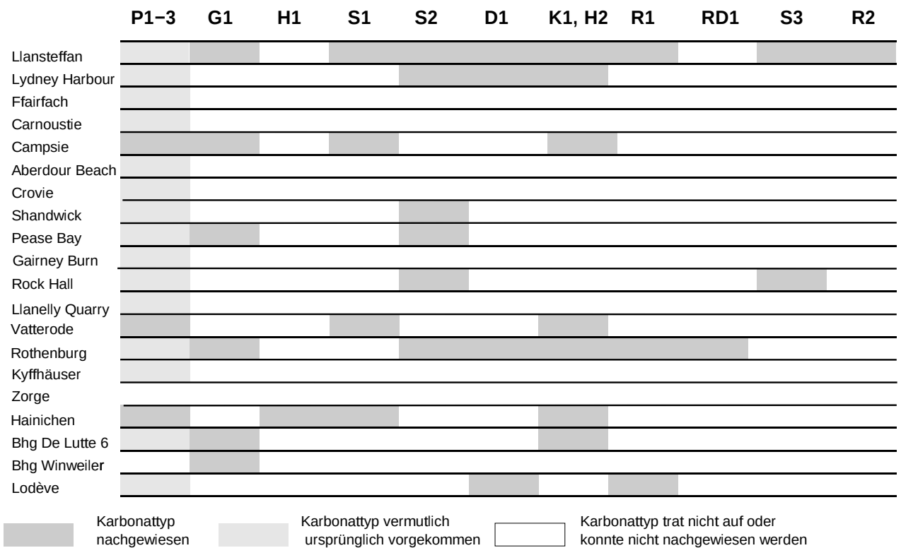
Abb. 20: Einordnung der untersuchten Lokalitäten in einen generalisierten Diageneseverlauf
