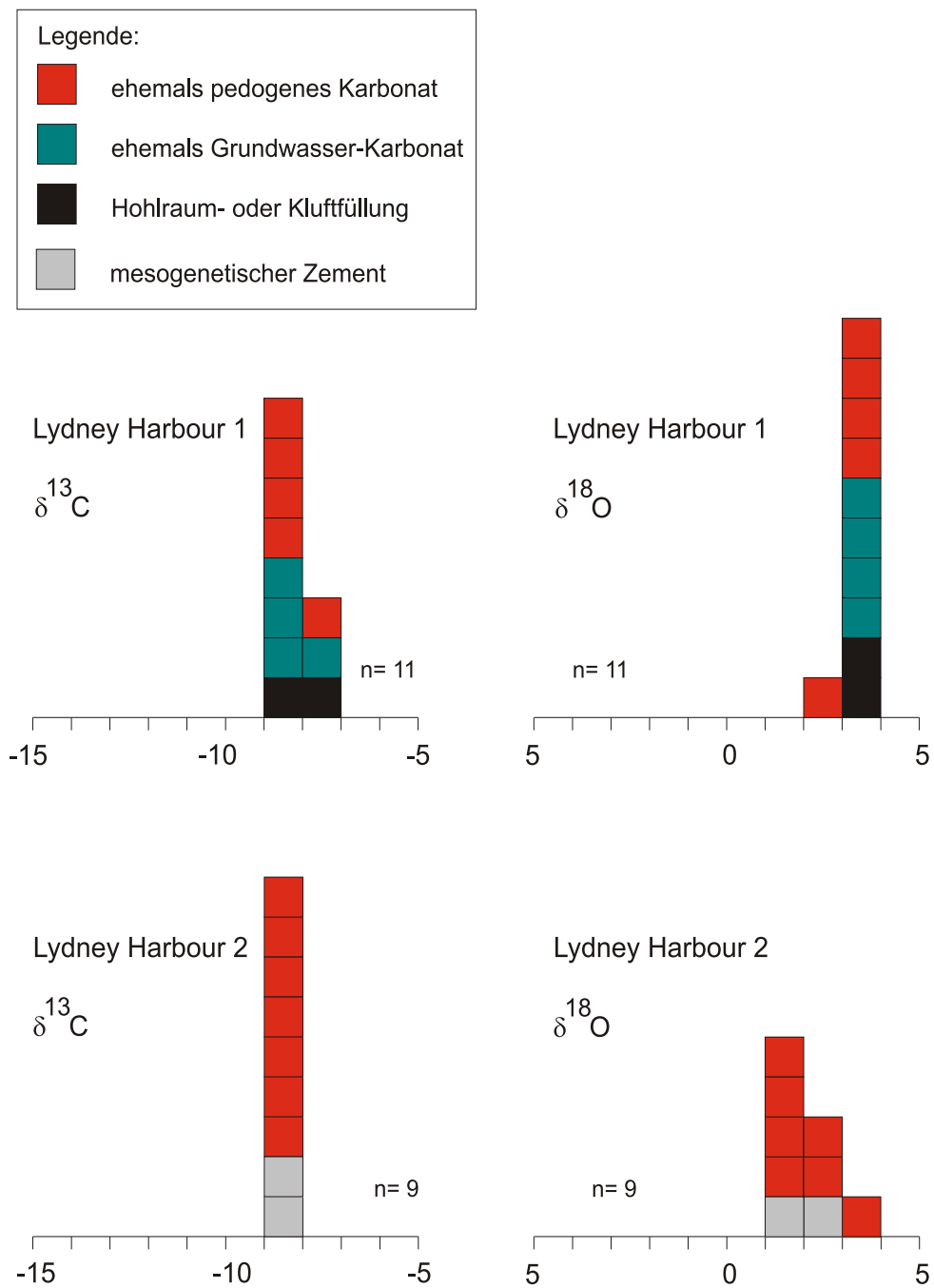
Abb. 22: Verteilung der C- und O-Isotopenwerte in den einzelnen Profilen der Lokalität Lydney Harbour.
